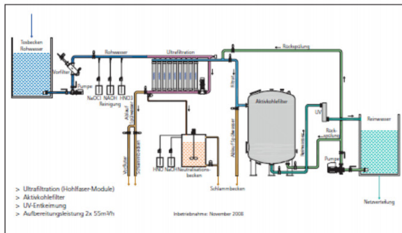
Abb. 1 Verfahrensschema der Aufbereitungsanlage Schönegg, Gemeinde Hergiswil.
